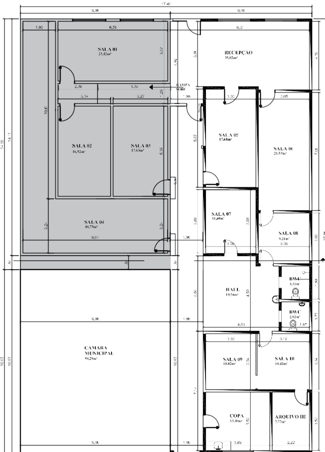
PLANTA BAIXA
